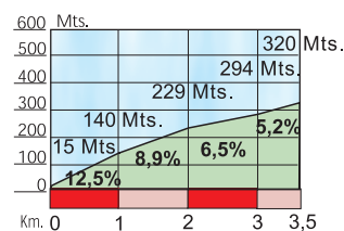
ALTO DE AIA 2ª Categoría Longitud: 3,5 Km. Pendiente media: 8,71%
