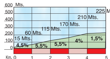
ALTO DE ITZIAR 3ª Categoría Longitud: 5 Km. Pendiente media: 4,2%
