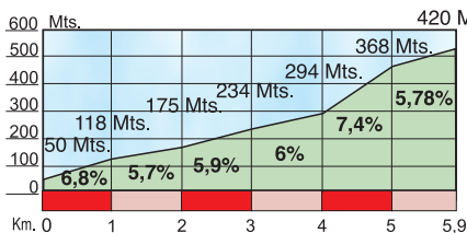
ALTO DE ANDAZARRATE 2ª Categoría Longitud: 5,9 Km. Pendiente media: 6,27%
