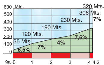
ALTO DE ALKIZA 2ª Categoría Longitud: 4,2 Km. Pendiente media: 6,79%
