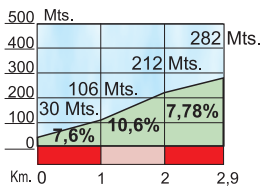
ALTO DE GARATE 2ª Categoría Longitud: 2,9 Km. Pendiente media: 8,69%
